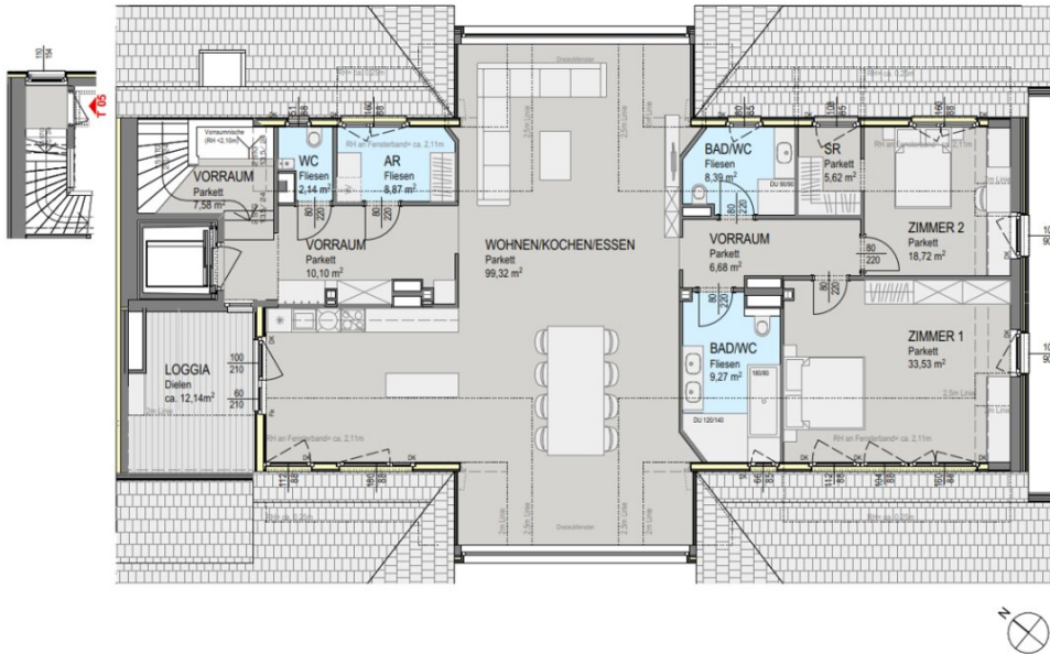
Grundriss Dachgeschoss
