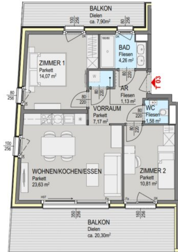
Grundriss Obergeschoss
