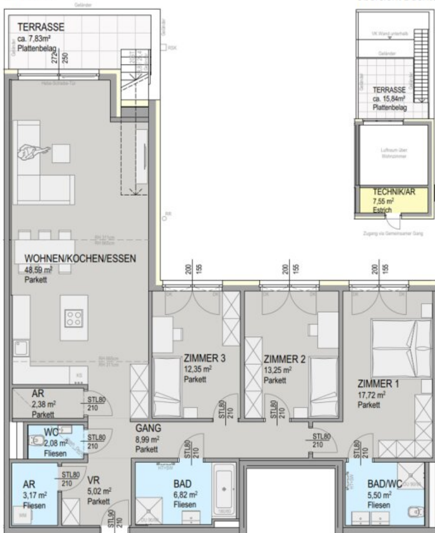
Grundriss:
