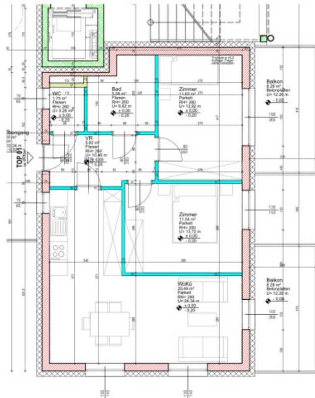
Planausschnitt 1.OBERGESCHOSS - Wohnung Planstand = Ausführungsplan M: 1:100
