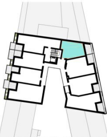
ORIENTIERUNGSPLAN | +4 OBERGESCHOSS
