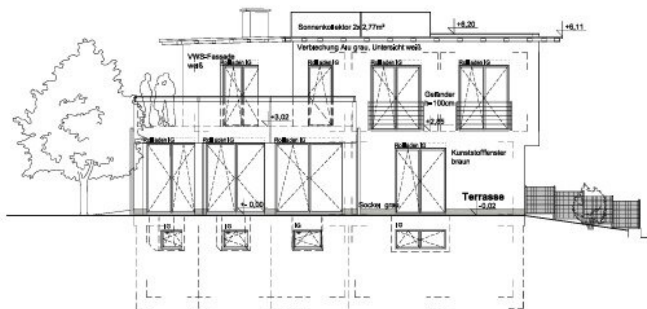
ANSICHT SÜDOST
