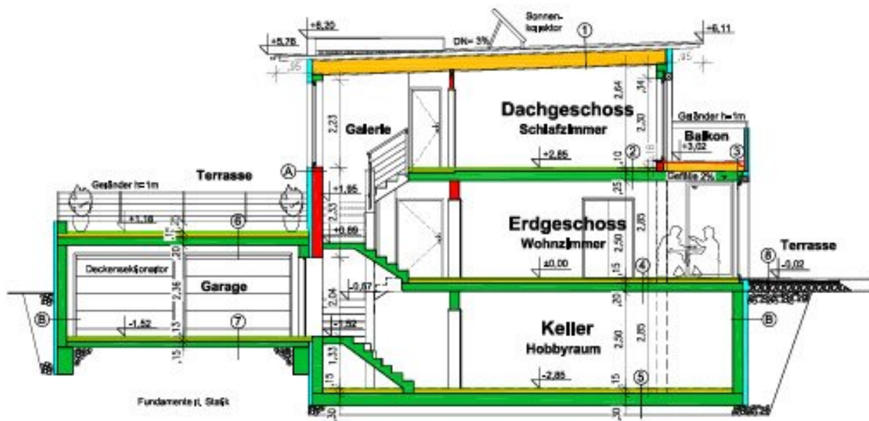
SCHNITT A-A
