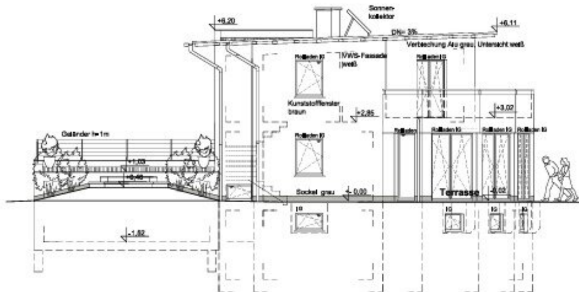
ANSICHT SÜDWEST
