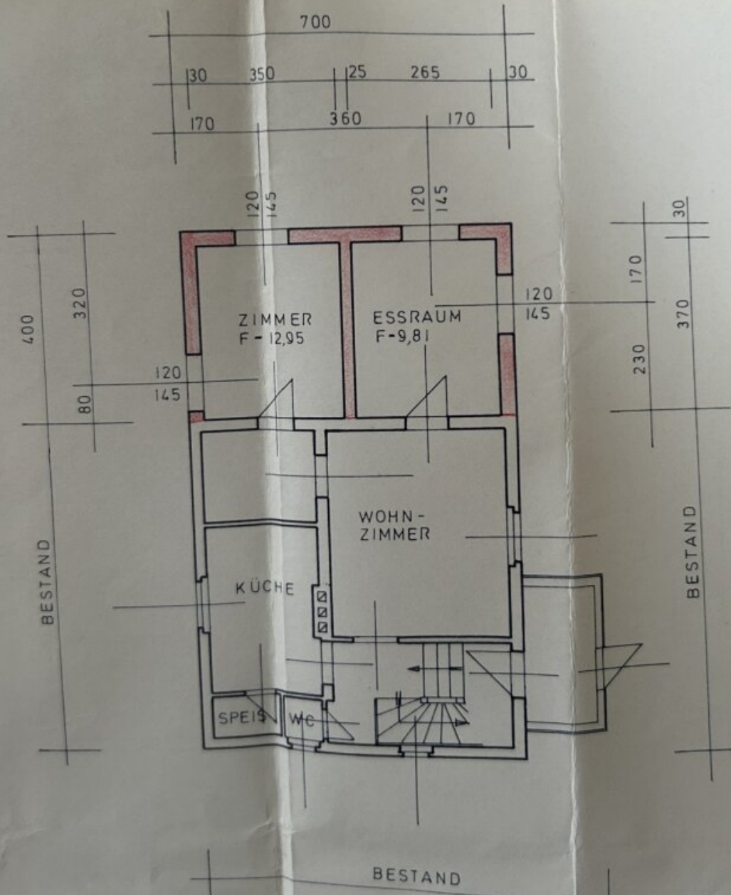
Planskizze Erdgeschoss
