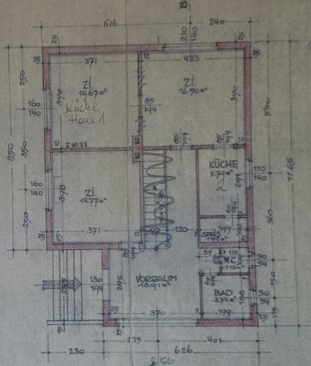
ERDGESCHOSS
