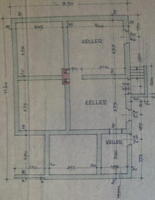
KELLERGESCHOSS
