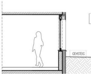
SCHNITT
