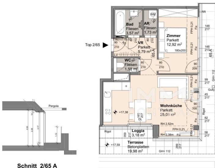
Schnitt 2/65 A
