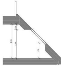
Schnitt 2/70 B
