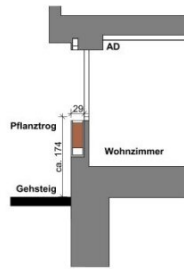
Fassadenschnitt
