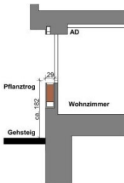
Fassadenschnitt
