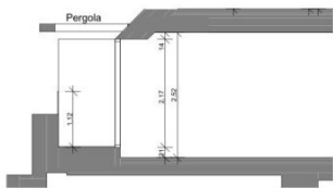
Schnitt 1/73 A
