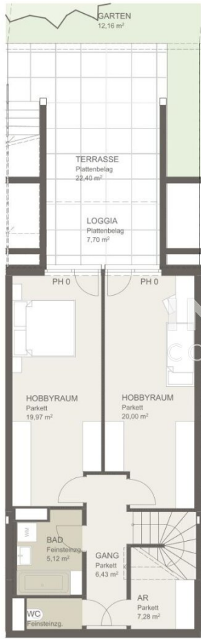
Untergeschoß
