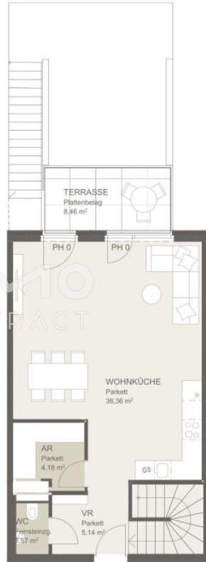
Erdgeschoß 8
