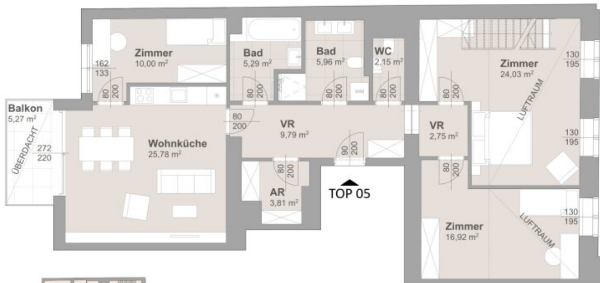
2. OBERGESCHOSS
