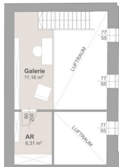
3. OBERGESCHOSS
