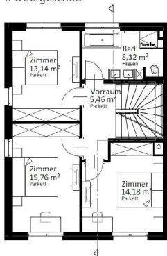
1. Obergeschoß
