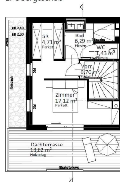
2. Obergeschoß
