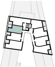
ORIENTIERUNGSPLAN | +1 OBERGESCHOSS
