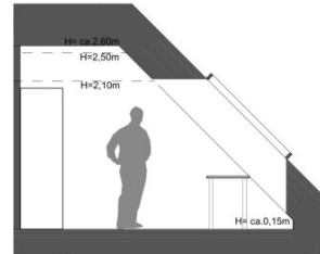
SCHNITT B
