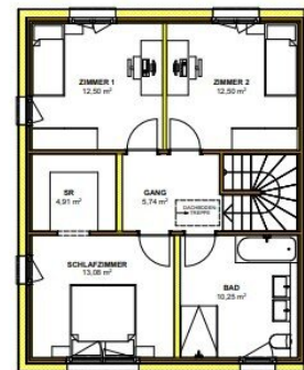
OBERGESCHOSS
