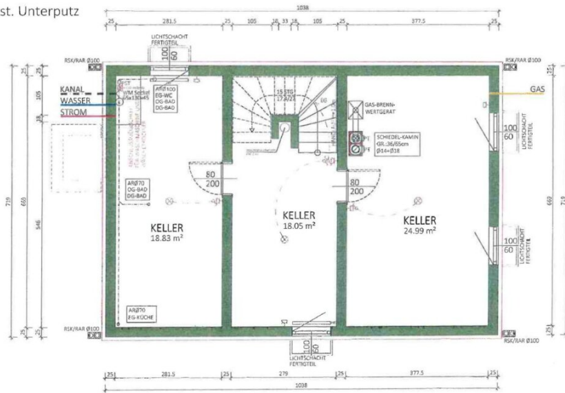
Kellergeschoss
