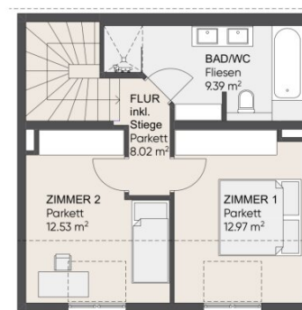
1. OG
