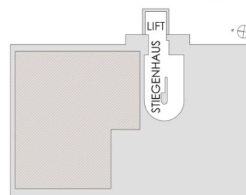
LAGEPLAN 1/250 GEIBELGASSE 24
