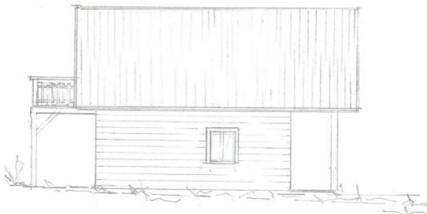
ANSICHT SÜD-WEST 1:100
