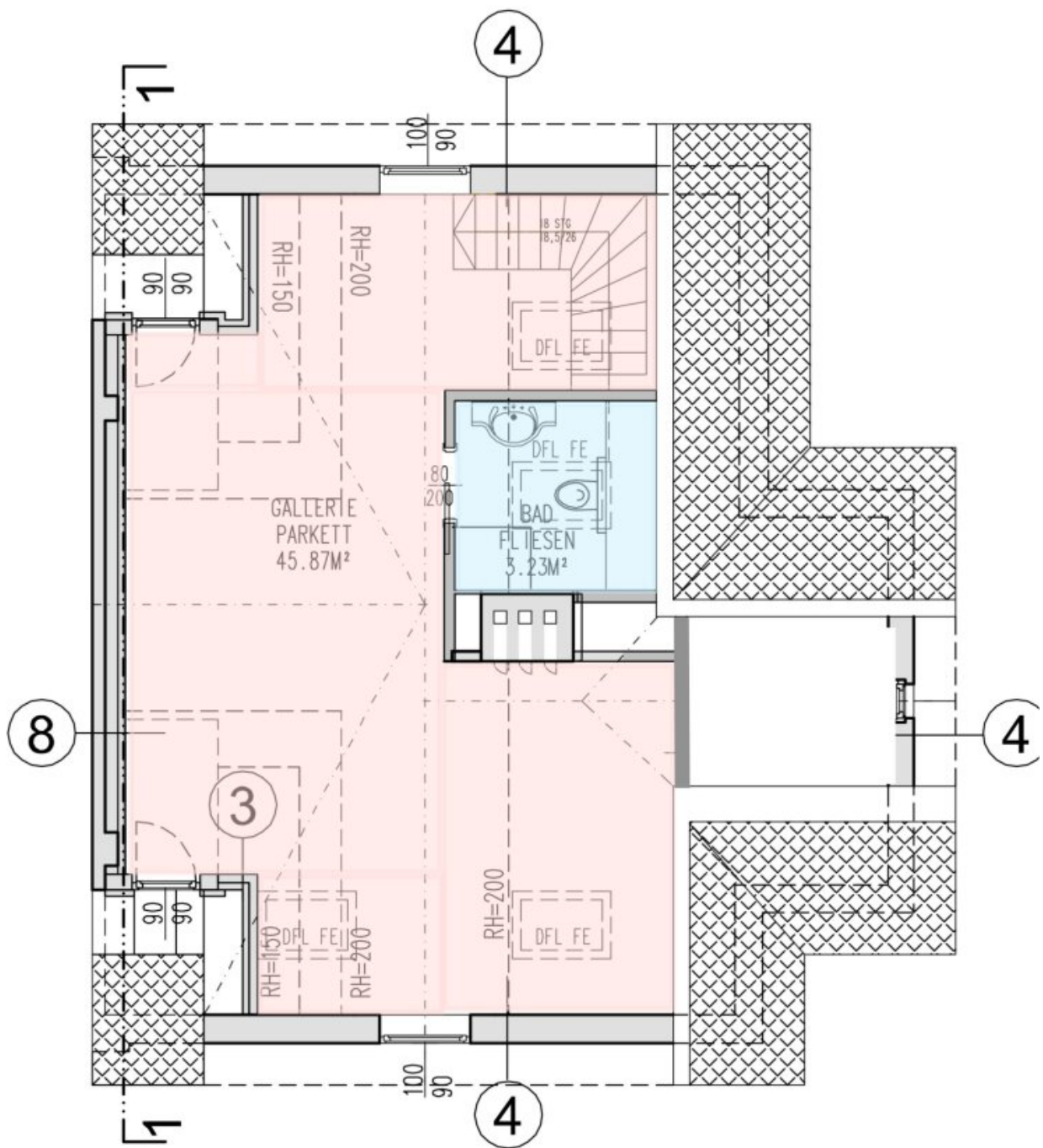
DACHGESCHOSS
