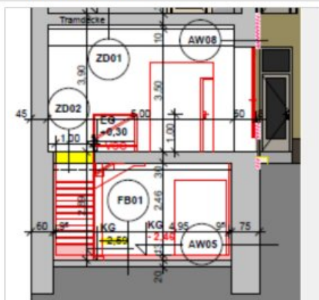
SCHNITT S05:
