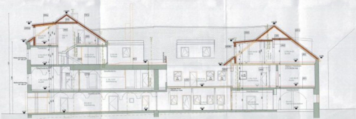
SCHNITT BB M1:100
