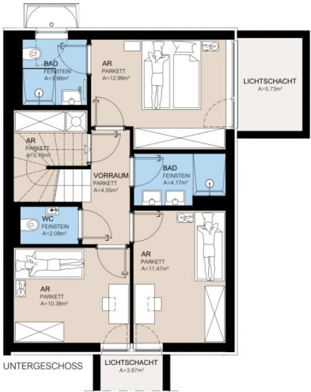
HAUS 01 TOP 01. UNTERGESCHOSS / ERDGESCHOSS
