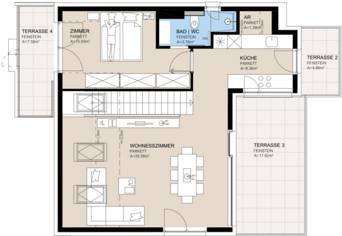
2. DACHGESCHOSS
