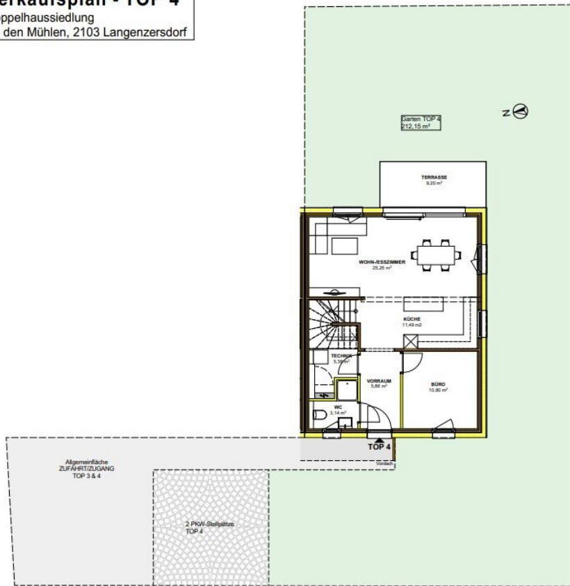
ERDGESCHOSS
