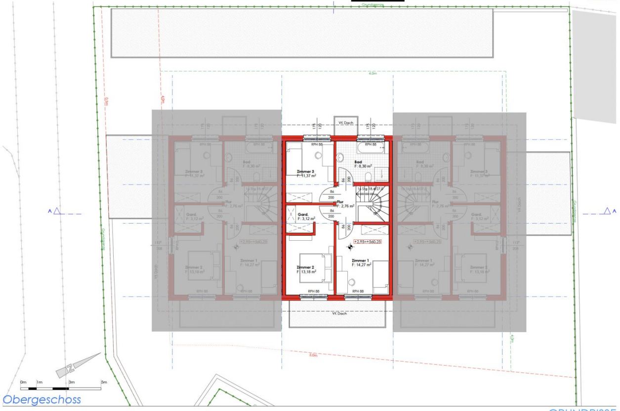
GRUNDRISS 1:100
