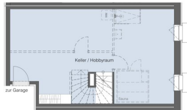
Kellergeschoss
