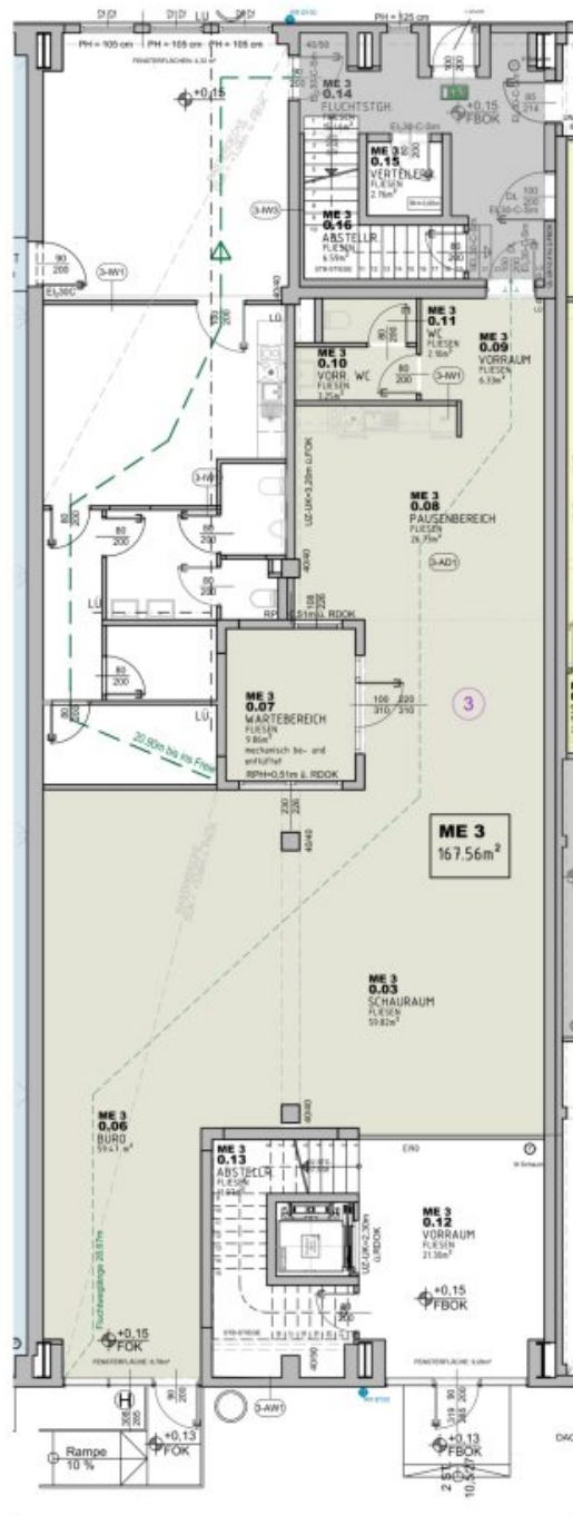
ERDGESCHOSS MIETEINHEIT 3
