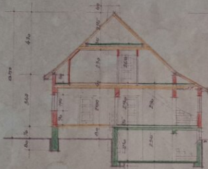
QUERSCHNITT
