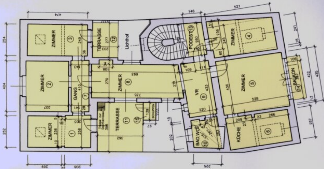
DACHGESCHOSS 1:100
