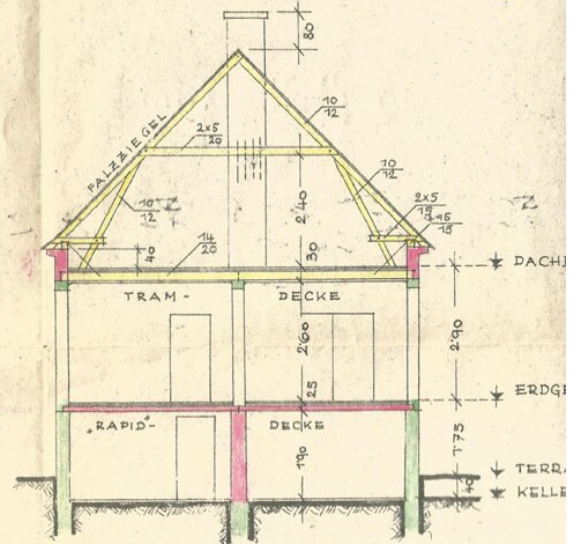
SCHNITT A-B
