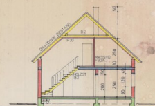
SCHNITT A-A
