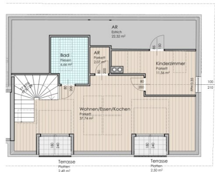
Grundriss DG
