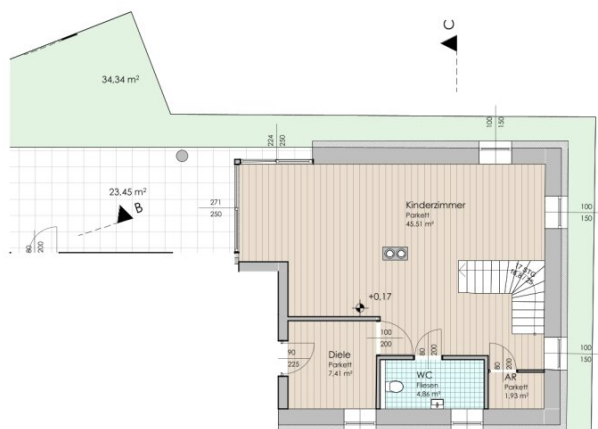
Grundriss EG
