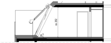
Schnitt 48.A
