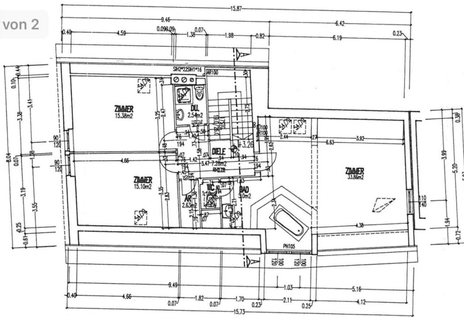
GRUNDRISZ DACHGESCHOSZ
