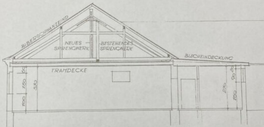
SNITT C-D
