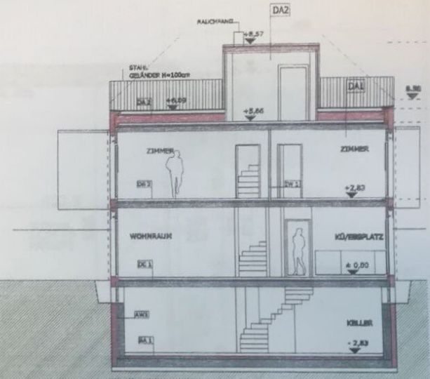
SCHNITT 1-1
