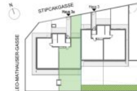
ÜBERSICHT ERDGESCHOSS
