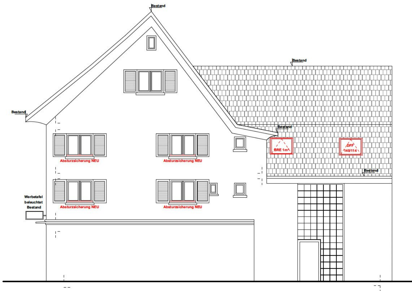
Nordansicht
