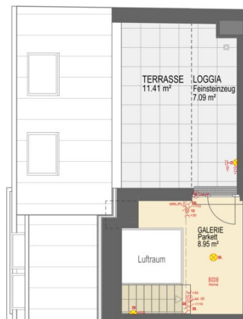
2. Dachgeschoss
