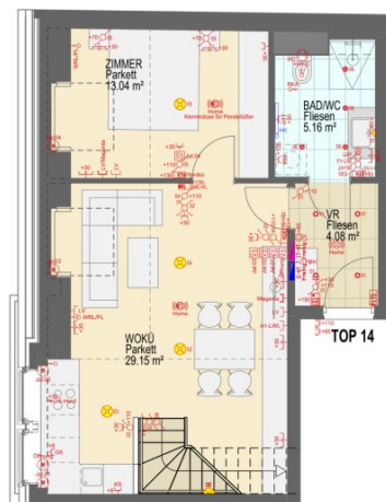
1. Dachgeschoss
