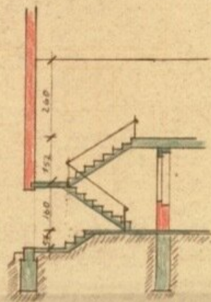
SCHNITT A-B
