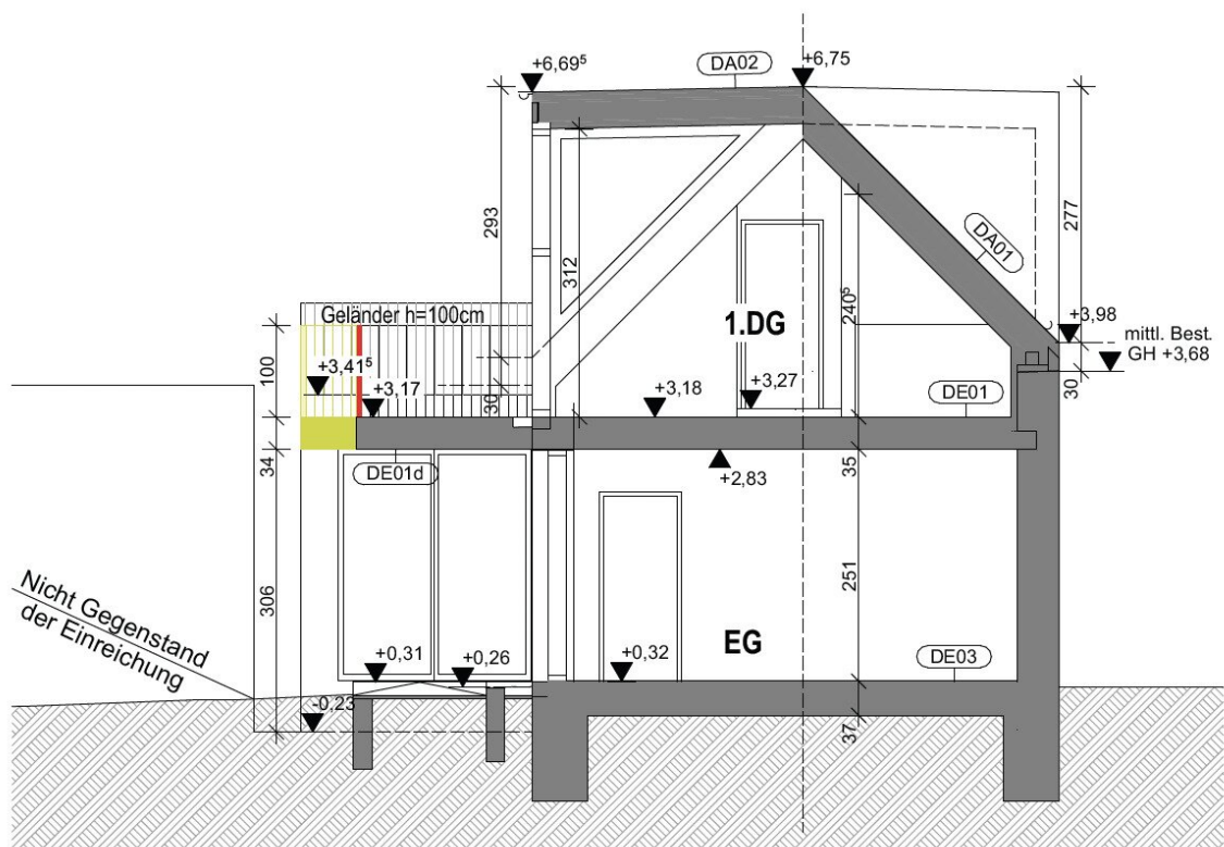
Schnitt A
