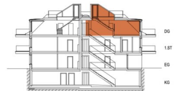
SCHNITT
