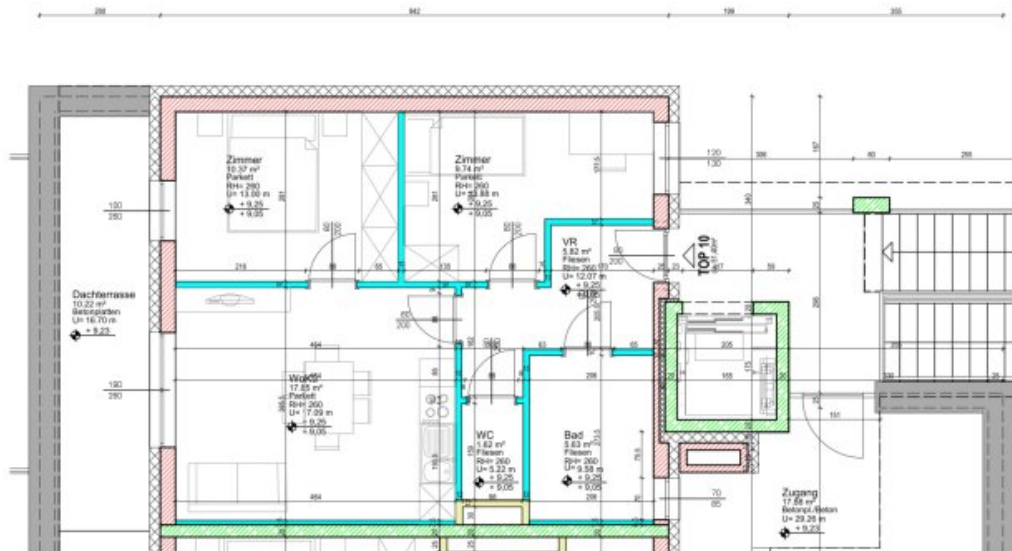
Planausschnitt 4.OBERGESCHOSS - Wohnung mit Dachterrasse Planstand = Ausführungsplan M: 1:100
