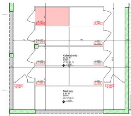
Planausschnitt KELLERGECHOSS - Abteil TOP 10 - OST Planstand = Ausführungsplan M: 1:100
